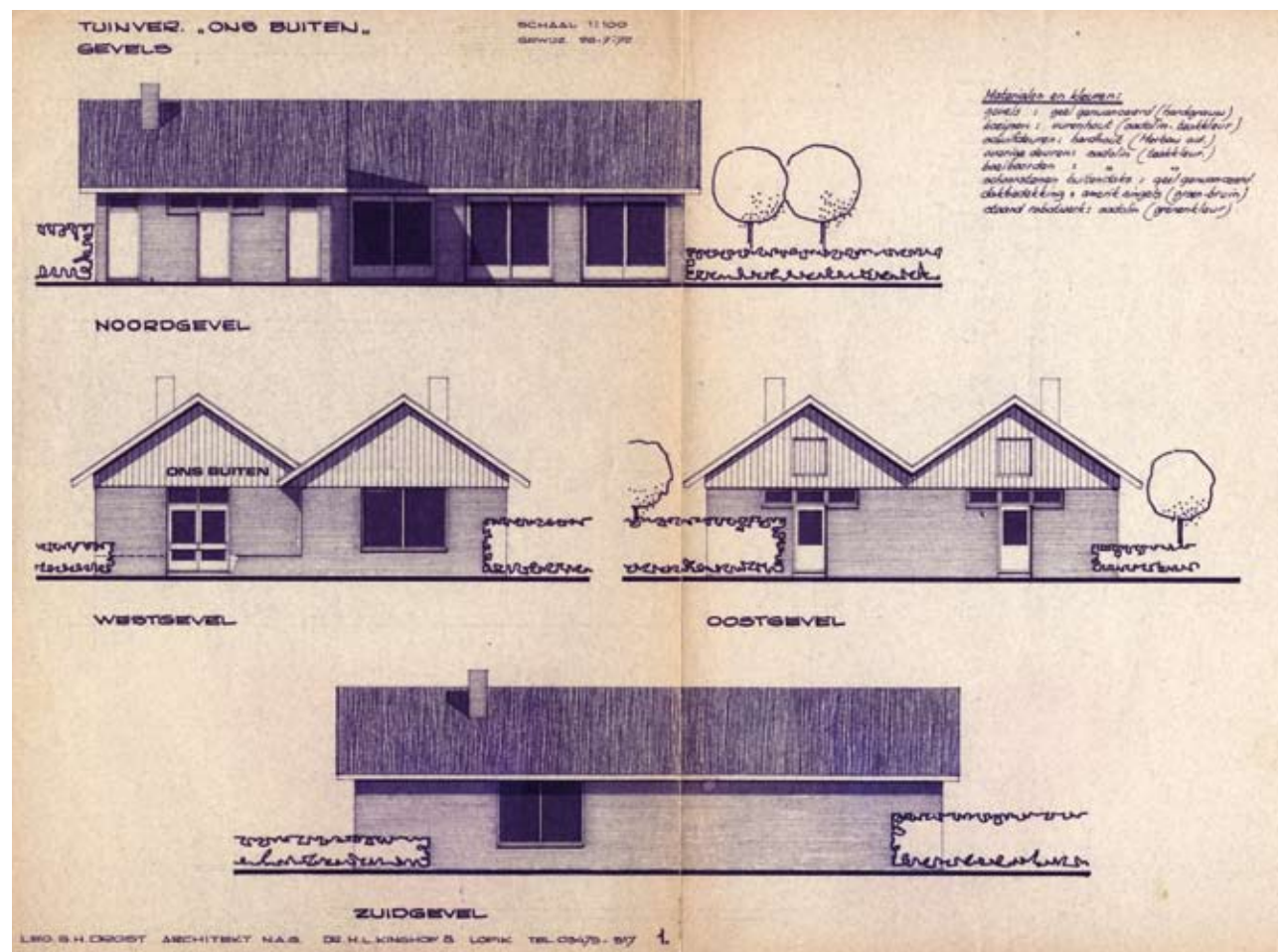
Bouwtekening van het in 1976 geopende clubhuis aan de toenmalige Lo Bruntlaan.
